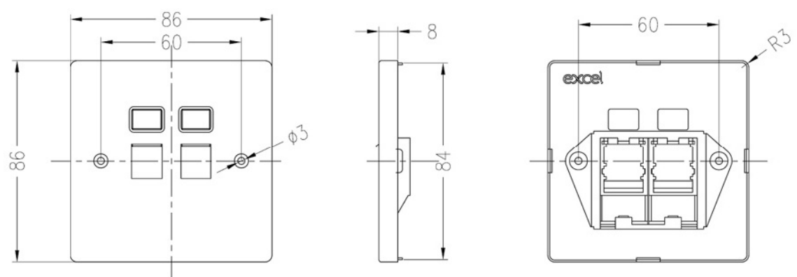
Dibujo del producto
