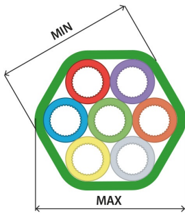
7-Way
