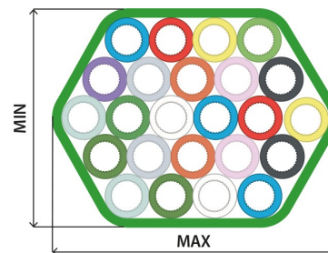
24-Way
